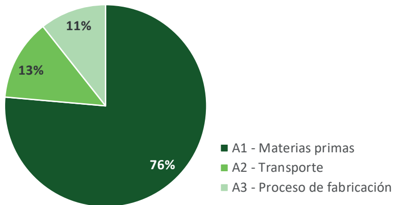
Potencial de calentamiento global (GWP) [kg CO 2 eq.] (1 kg de sistema de tuberías FASER)
