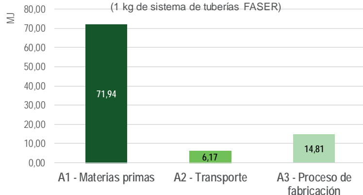
Fuentes de energía primarias (MJ) (1 kg de sistema de tuberías FASER)
