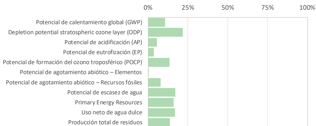
Evaluación de la etapa A3 (Proceso de fabricación) sobre la etapa total de producción (A1 + A2 + A3) para el desempeño ambiental, el uso de agua y la producción de desechos (1 kg de sistema de tuberías FASER)
