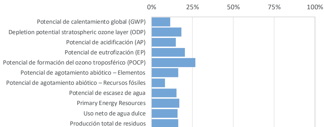
Evaluación de la etapa A3 (Proceso de fabricación) sobre la etapa total de producción (A1 + A2 + A3) para el desempeño ambiental, el uso de agua y la producción de desechos (1 kg de sistema de tuberías ENERGY)
