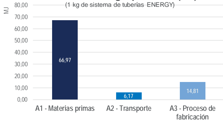
Fuentes de energía primarias (MJ) (1 kg de sistema de tuberías ENERGY)
